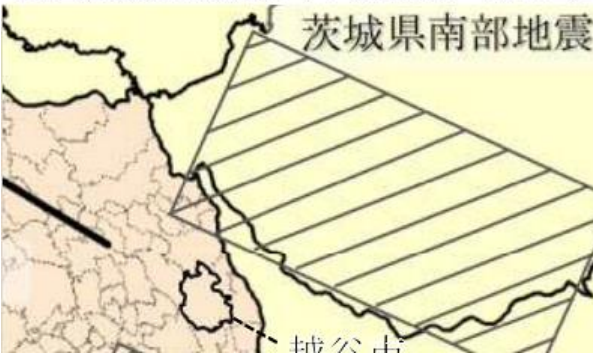
●埼玉県地震被害想定調査における想定地震の断層位置図
